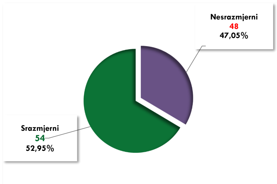
Grafikon 7: Grafički prikaz utvrđenog (ne)srazmjera u do sada 102 okončane provjere
